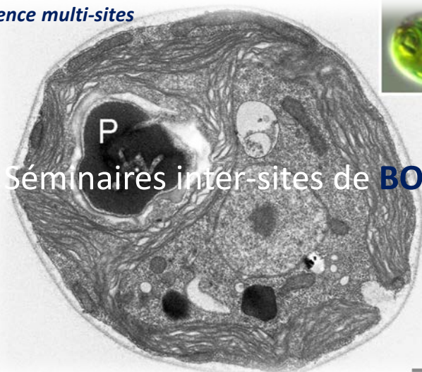
Micrographie de l'algue unicellulaire Chlamydomonas reinhardtii (en vignette, image en microscopie optique ; P : pyrénoïde ; échelle : 1 micron). © M. Meyer.
